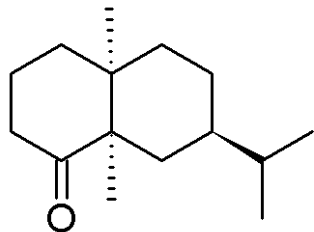
valeranon
