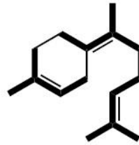
bisabolen
