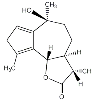
ahilicin (8-acetilartabsin)
