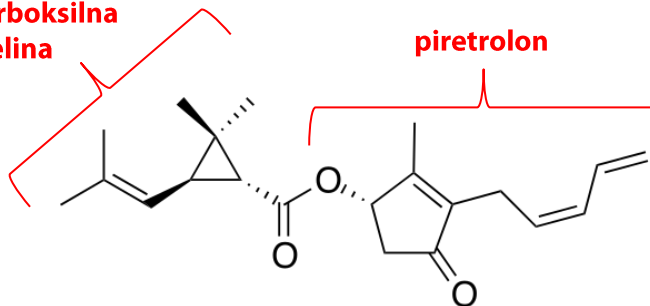
piretrin I
