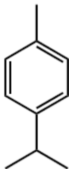
p -cimen
