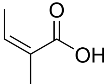
angelinska kiselina
