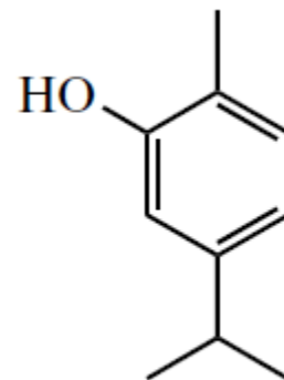
karvakrol
