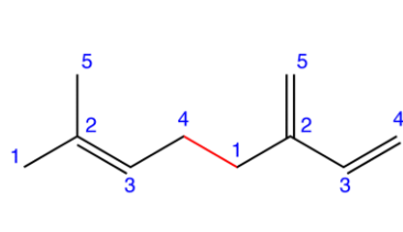
mircen
