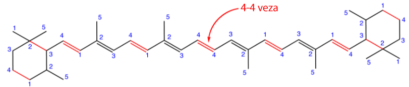
\beta -karoten
